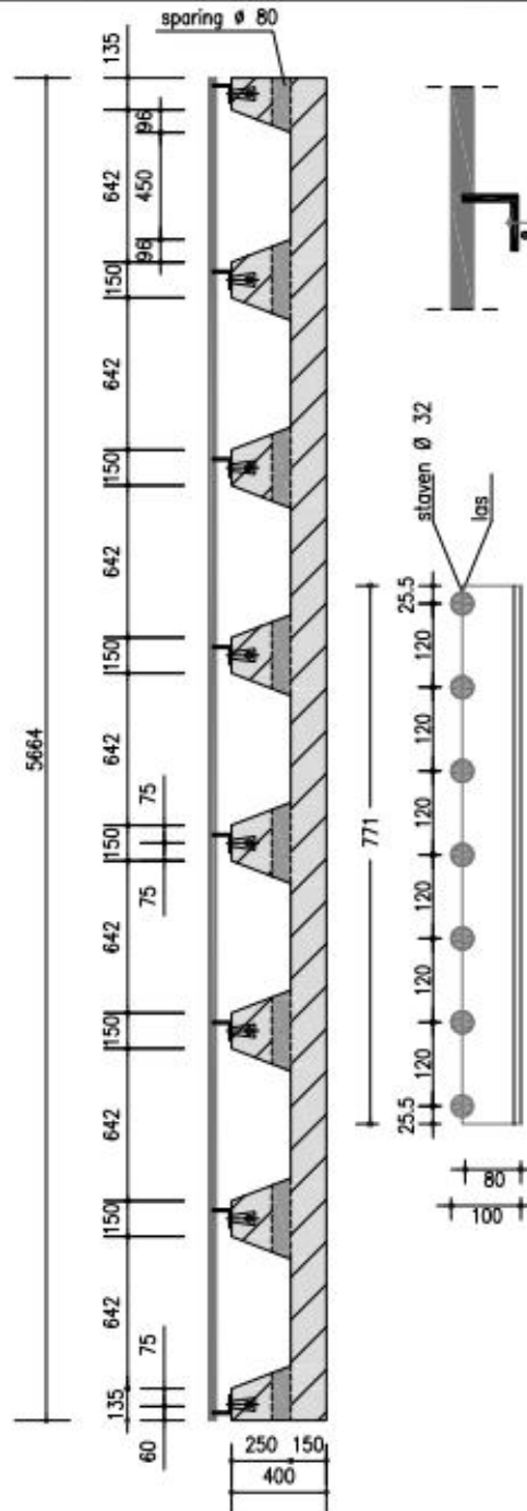
Langsdoorsnede
