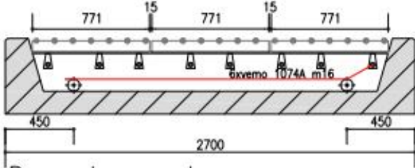
Dwarsdoorsnede
