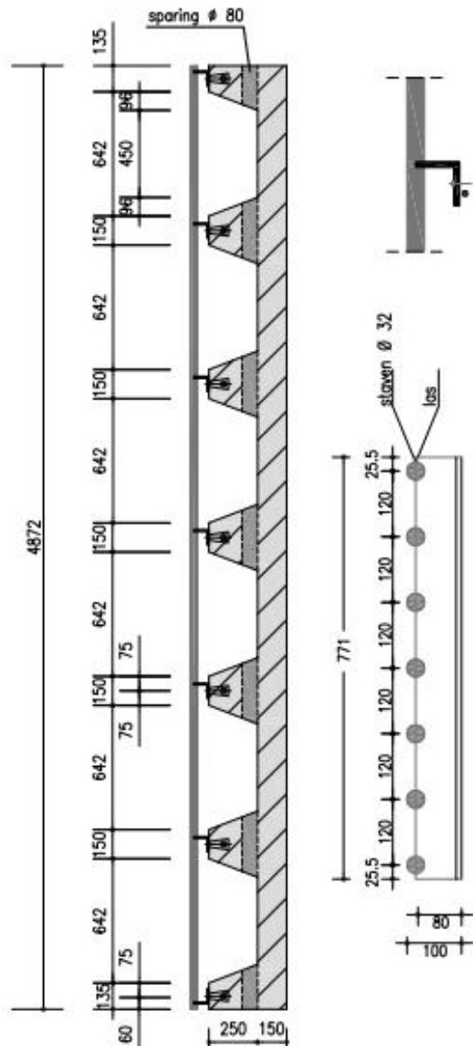
Langsdoorsnede
