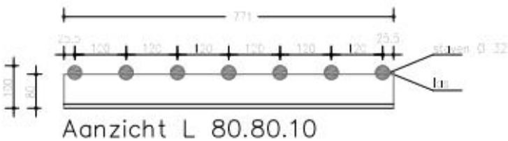
Dwarsdoorsnede
