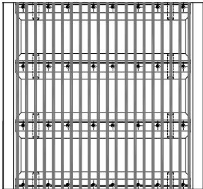
Bovenaanzicht
