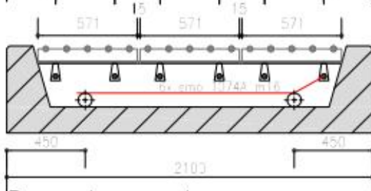
Dwarsdoorsnede
