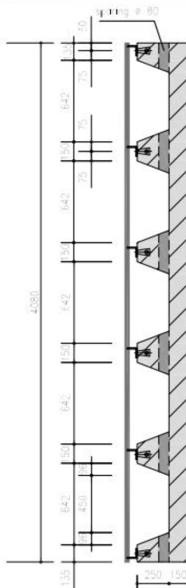
Langsdoorsnede
