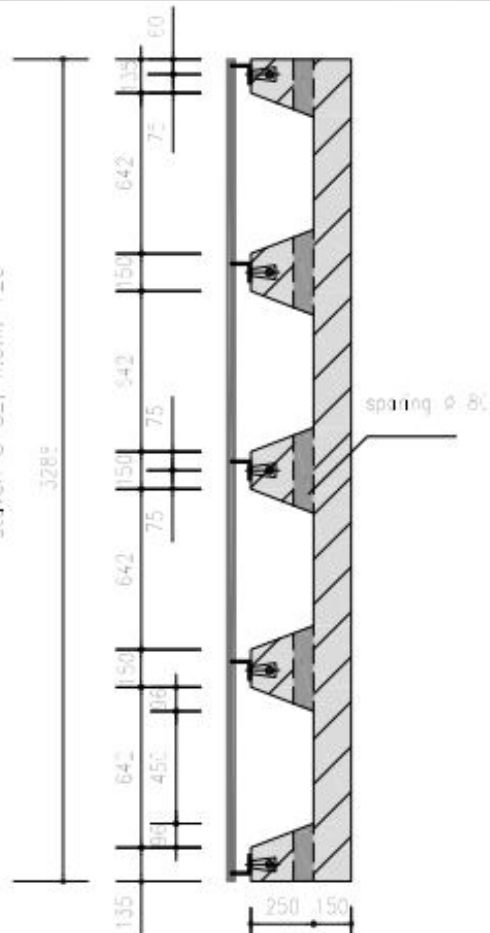
Langsdoorsnede
