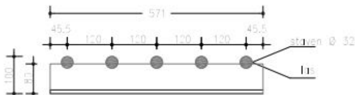
Aanzicht L 80.80.10
