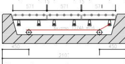
Dwarsdoorsnede
