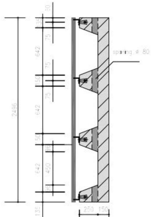
Langsdoorsnede
