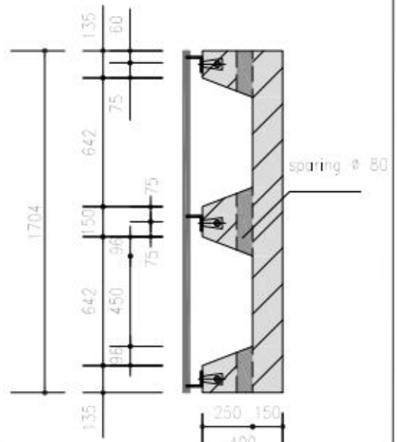
Langsdoorsnede
