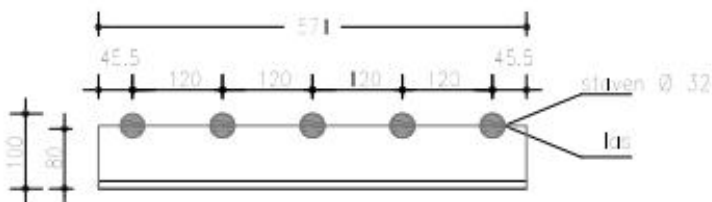
Aanzicht L 80.80.10
