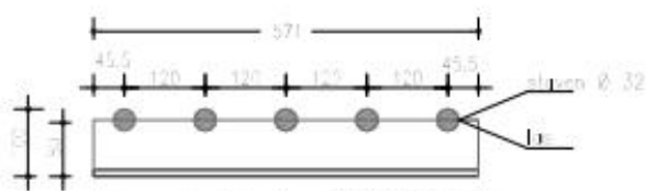
Aanzicht L 80.80.10
