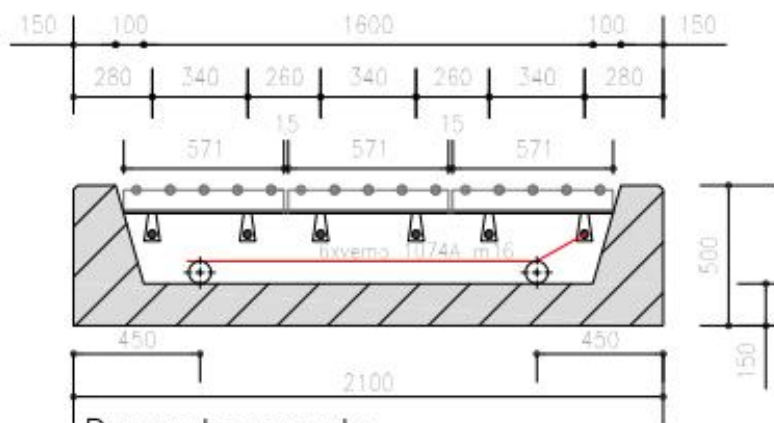
Dwarsdoorsnede
