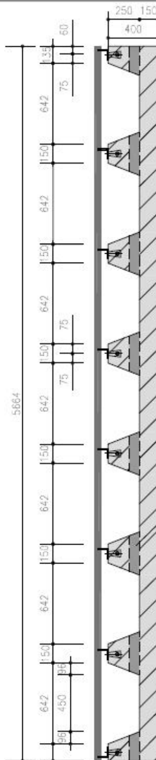
Langdoorsnede
