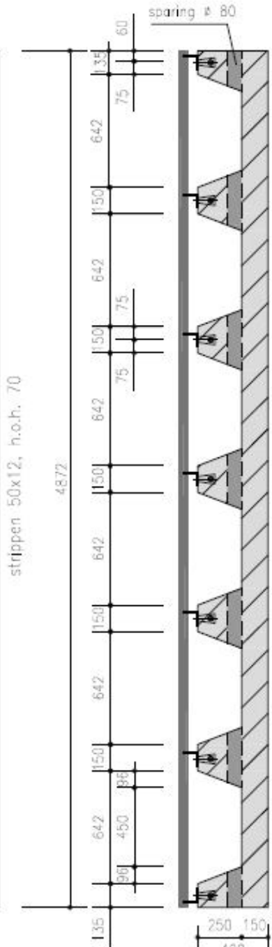
Langdoorsnede
