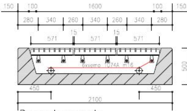
Dwarsdoorsnede
